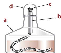
Fig. 1.18. Părțile componente ale spirtierei: a – vas pentru alcool; b – tub cu disc; c – fitil; d – capac
