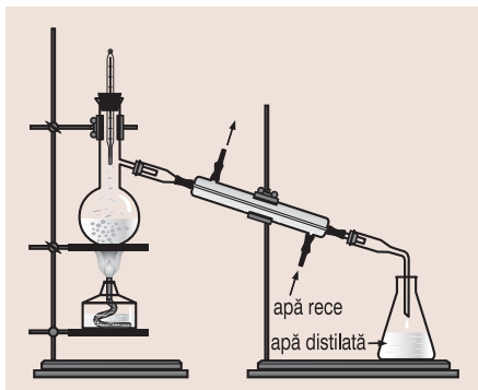
Fig. 4.7. Distilarea apei naturale într-o instalație de laborator
