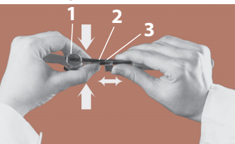
Fig. 1.16. Clemă pentru eprubete: 1 – eprubetă; 2 – plăci metalice; 3 – colier
