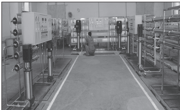
Fig. 4.8. Distilarea apei naturale într-o instalație industrială
