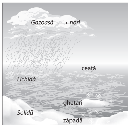
Fig. 4.12. Stările de agregare ale apei în natură
