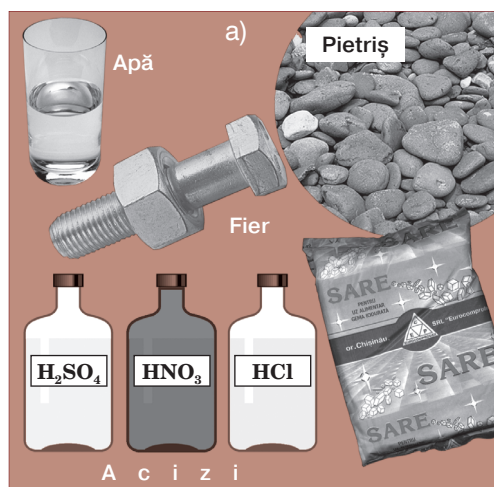
Fig. 1.7. Substanțe și materiale: a) anorganice; b) organice
