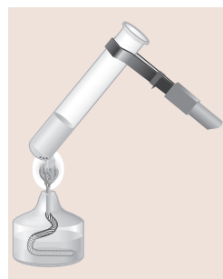
Fig. 1.21. Încălzirea substanțelor lichide
