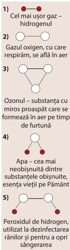
Fig. 3.1. Formarea diferitor substanțe din atomii a două elemente – hidrogenul ● și oxigenul ○
