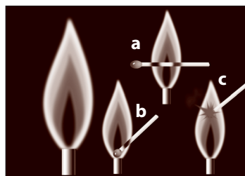
Fig. 1.20. Arderea chibritului în diferite părți ale flăcării
