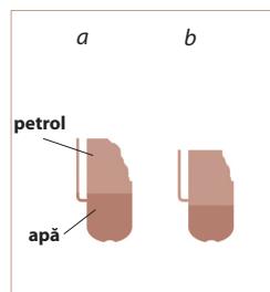
Fig. 4.4. Coloană de separare: a – scurgerea apei; b – scurgerea petrolului
