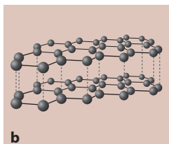
Fig. 3.2. Aranjarea atomilor de carbon în cristalele de: a – diamant, b – grafit
