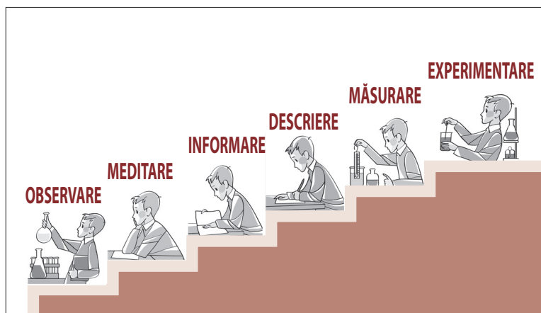
Fig. 1.13. Consecutivitatea metodelor de cunoaștere în chimie
