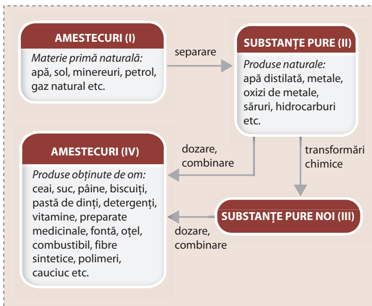
Fig. 4.1. Importanța amestecurilor și a substanțelor pure în crearea produselor și materialelor necesare omului
