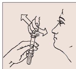
Fig. 1.24. Stabilirea mirosului unei substanțe chimice
