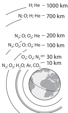
Fig. 4.17. Compoziția învelișului gazos al Pământului la diferite înălțimi
