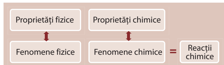
Fig. 1.29. Corelația proprietăți – fenomene
