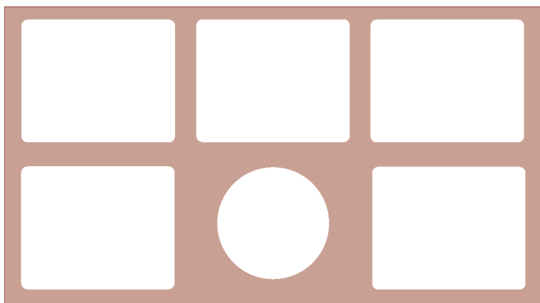
Fig. 4.18. Surse de poluare a mediului
