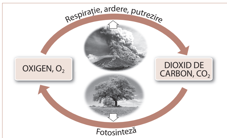
Fig. 4.16. Procesul natural reversibil de consumare a oxigenului și de regenerare a lui prin fotosinteză
