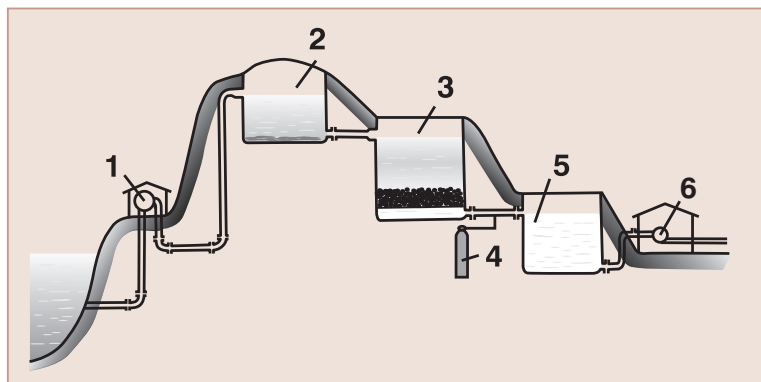
Fig. 4.15. Schema stației de epurare a apei: 1 – pompă; 2 – bazin de decantare; 3 – filtru; 4 – dispozitiv pentru clorurare sau tratarea cu hipoclorit de sodiu a apei; 5 – bazin de limpezire; 6 – pomparea apei spre consumator.
