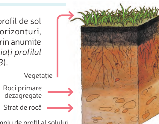
Fig. 3.18. Exemplu de profil al solului
