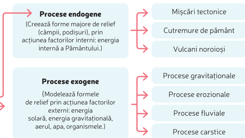
Fig. 1.15. Clasificarea proceselor de modelare a reliefului
