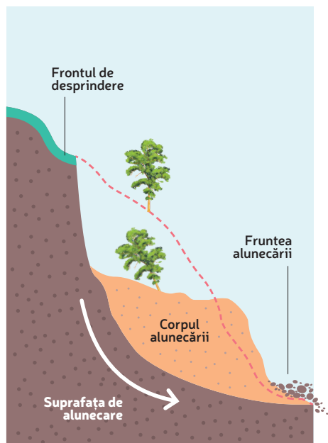
Fig. 1.25. Elementele unei alunecări de teren
