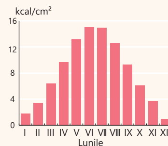
Fig. 2.1. Valorile lunare ale radiației solare globale. Stația Meteorologică Chișinău
