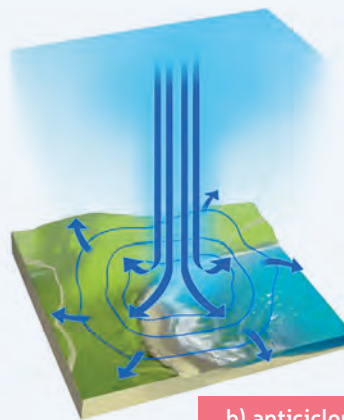
b) anticiclon
