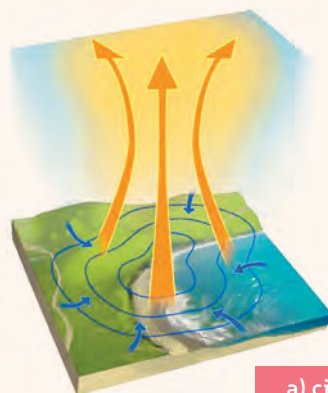
a) ciclon
